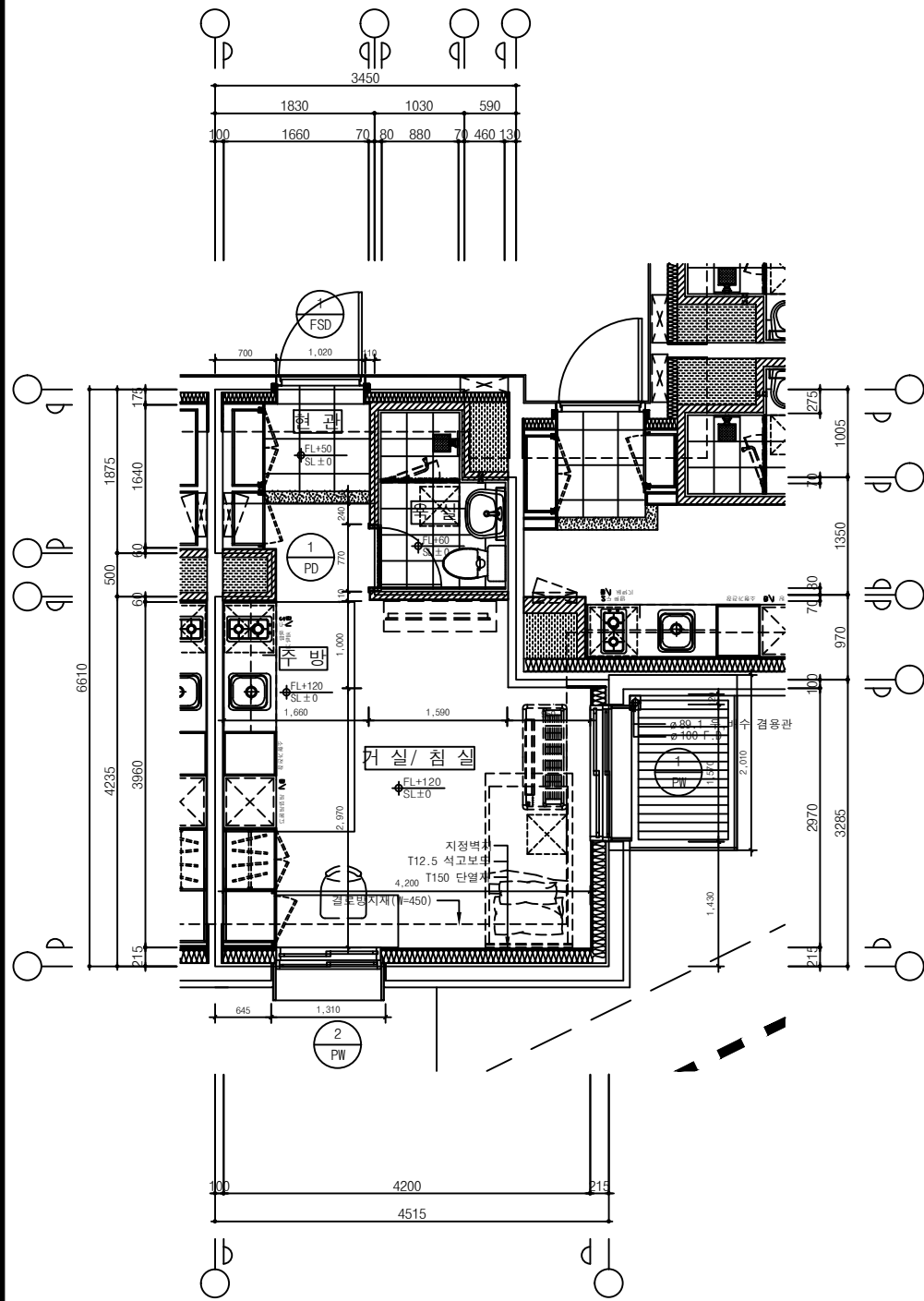
3 22m² 형 단위세대 평면도(C-type) SCALE : A1 : 1/40 A3 : 1/80
