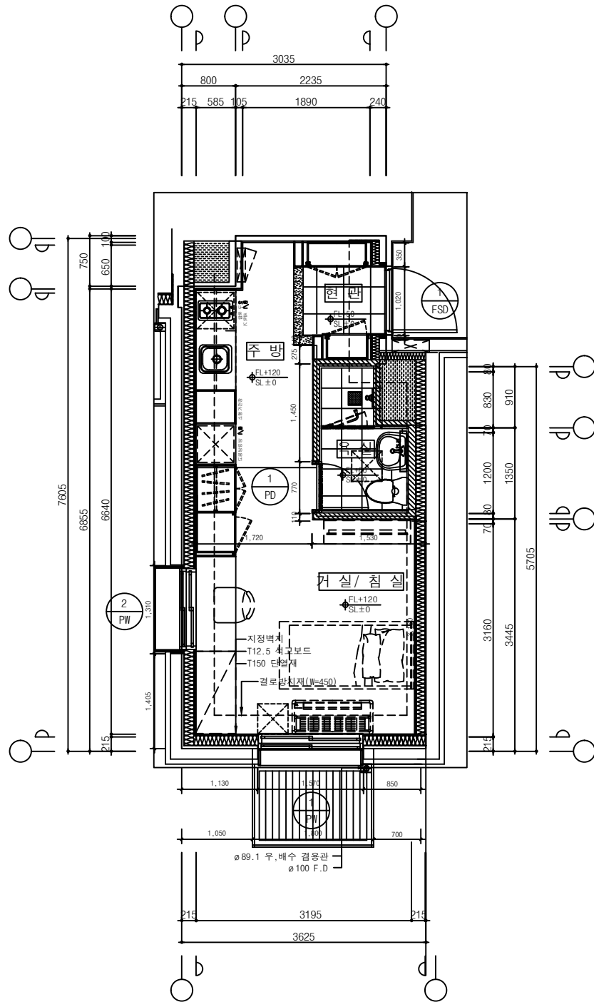
4 A 21㎡형 단위세대 평면도(D-1type)4,5 층 SCALE : A1 : 1/40 A3 : 1/80
