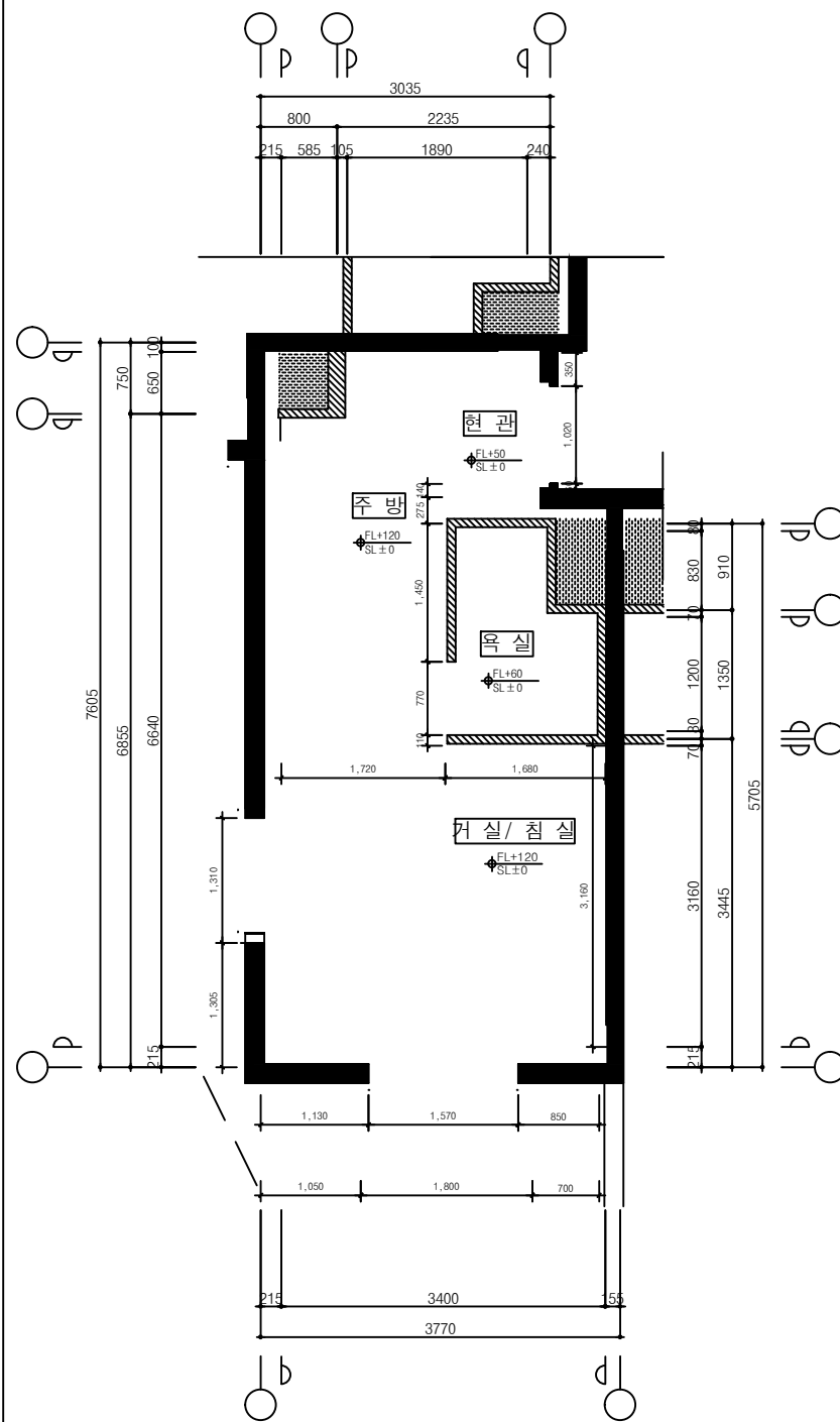
4 22m² 형 단위세대 평면도(D-type) SCALE : A1 : 1/40 A3 : 1/80
