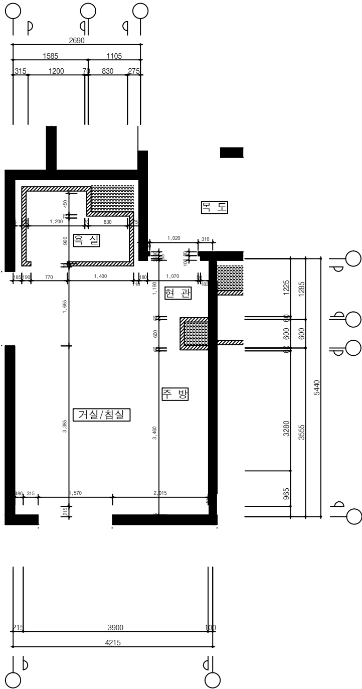
1 22m² 형 단위세대 평면도(A-type)
