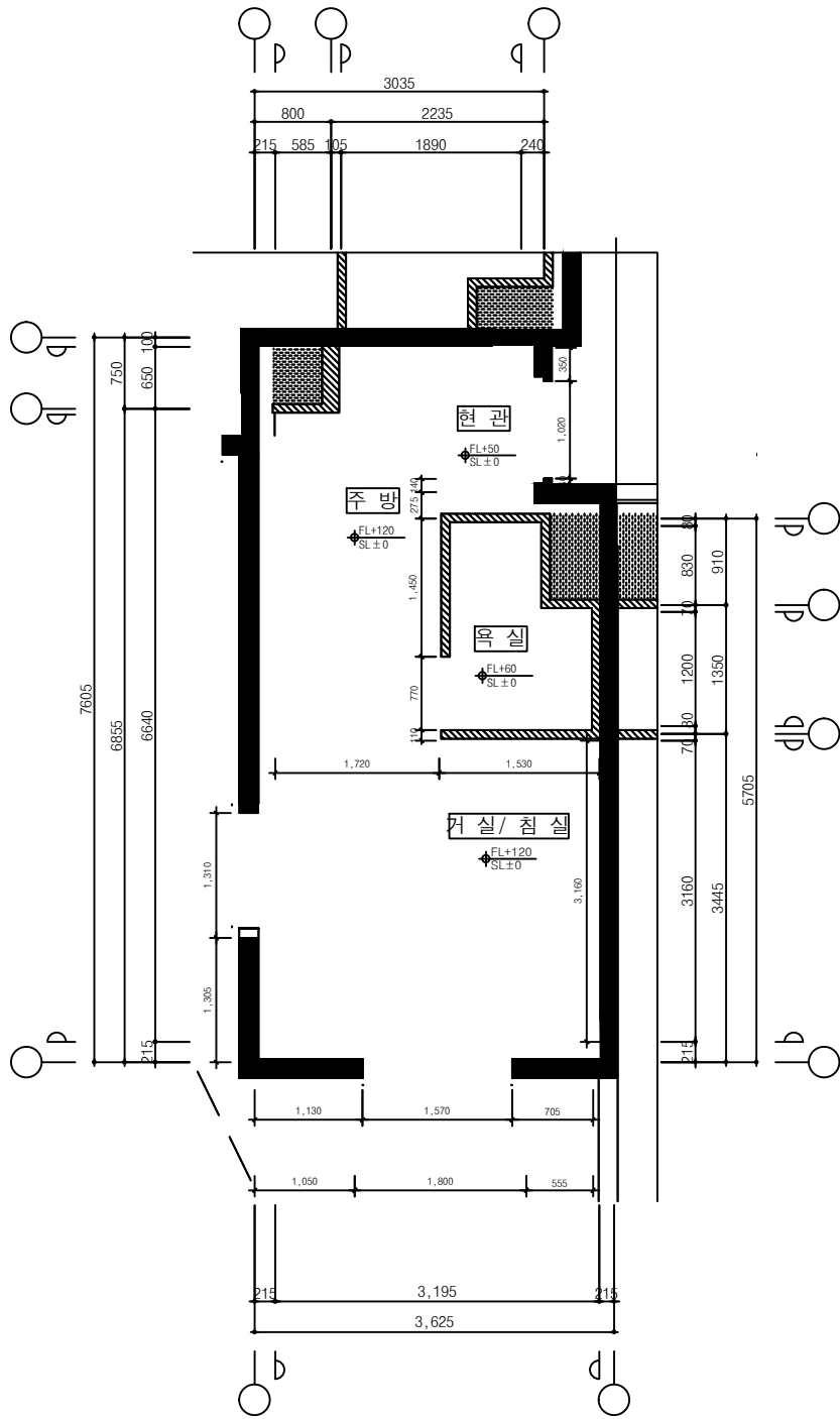
4 21㎡형 단위세대 평면도(D-1type)4,5층 A SCALE : A1 : 1/40 A3 : 1/80
