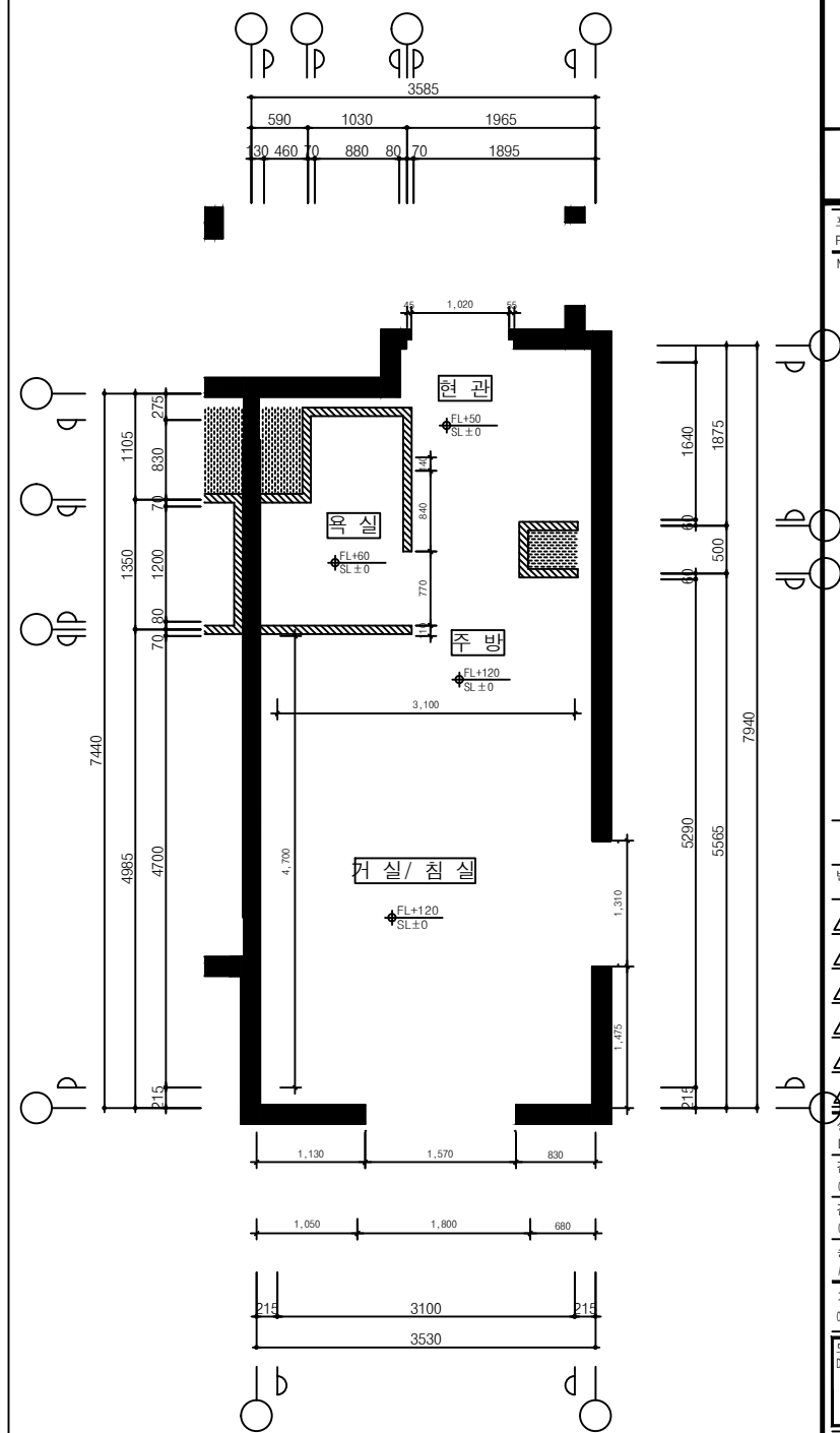
5 22m² 형 단위세대 평면도(E-type) SCALE : A1 : 1/40 A3 : 1/80
