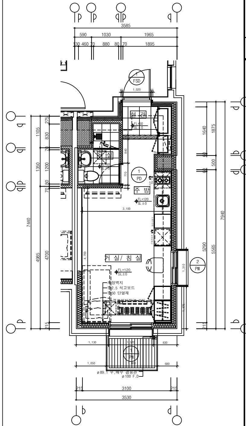
5 22m² 형 단위세대 평면도(E-type) SCALE : A1 : 1/40 A3 : 1/80
