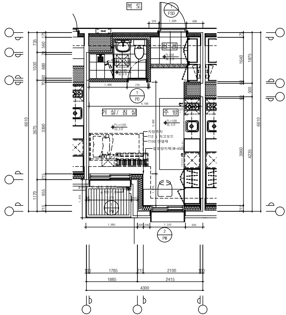
2 22m² 형 단위세대 평면도(B-type) SCALE : A1 : 1/40 A3 : 1/80
