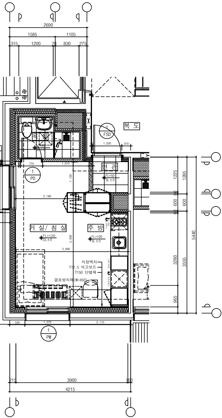
1 22m² 형 단위세대 평면도(A-type) SCALE : A1 : 1/40 A3 : 1/80
