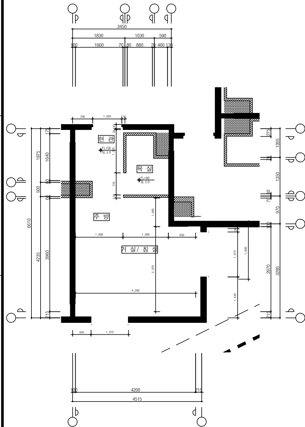
3 22m² 형 단위세대 평면도(C-type) SCALE : A1 : 1/40 A3 : 1/80
